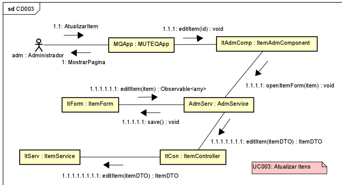
Figura 49. Diagrama de comunicação para o [UC003].
