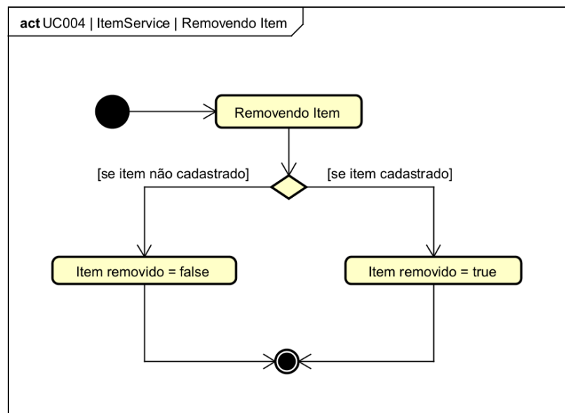
Figura 106. Diagrama de Atividades do estado “Removendo Item” da classe ItemService para o [UC004].
