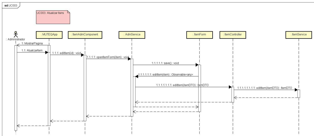
Figura 32. Diagrama de sequência para o [UC003].
