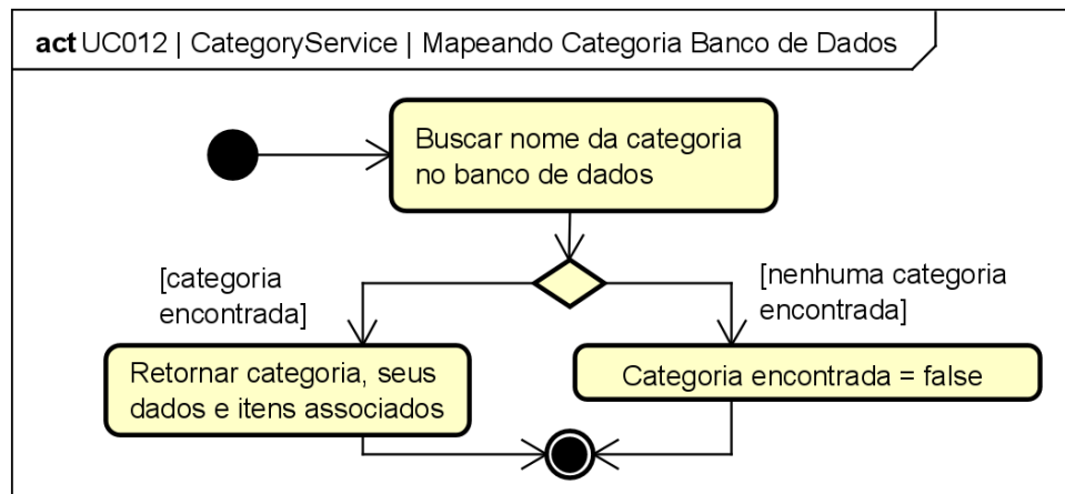
Figura 121. Diagrama de Atividades do estado “Mapeando Categoria Banco de Dados” da classe CategoryService para o [UC012].
