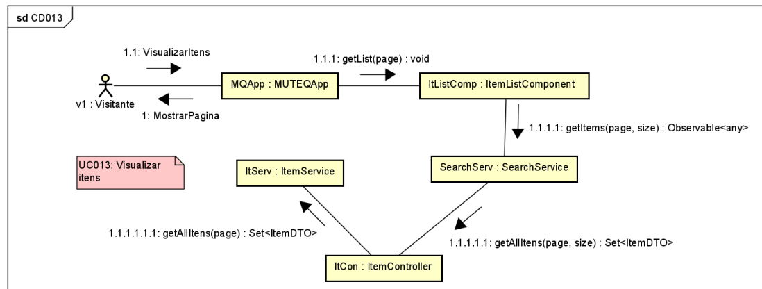
Figura 59. Diagrama de comunicação para o [UC013].
