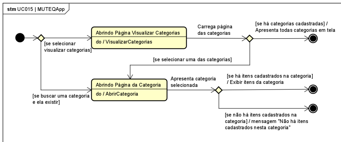
Figura 93. Diagrama de Estados da classe MUTEQApp para o [UC015].
