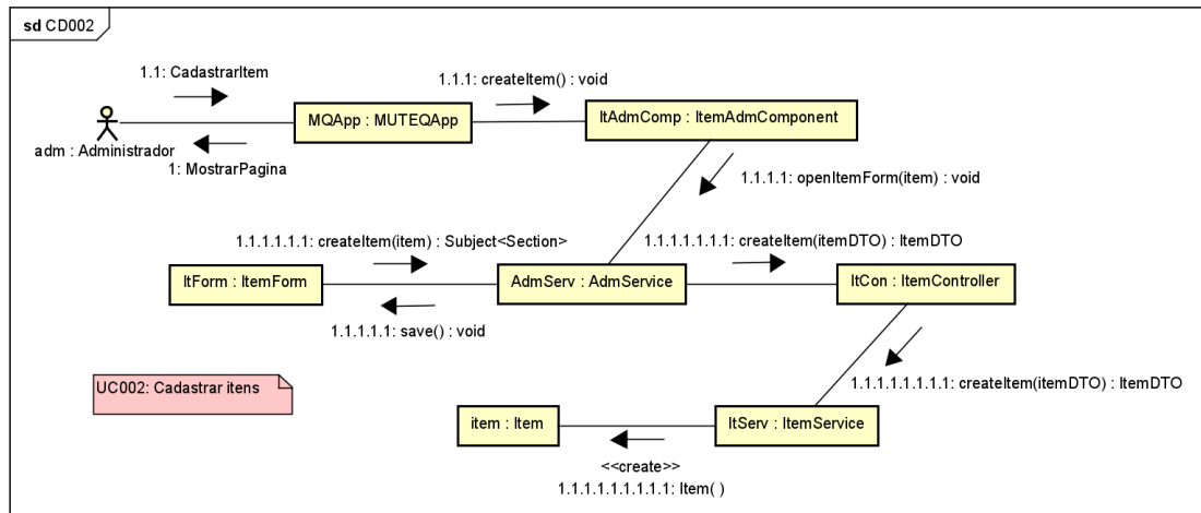
Figura 48. Diagrama de comunicação para o [UC002].
