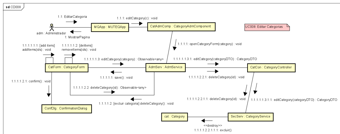
Figura 54. Diagrama de comunicação para o [UC008].
