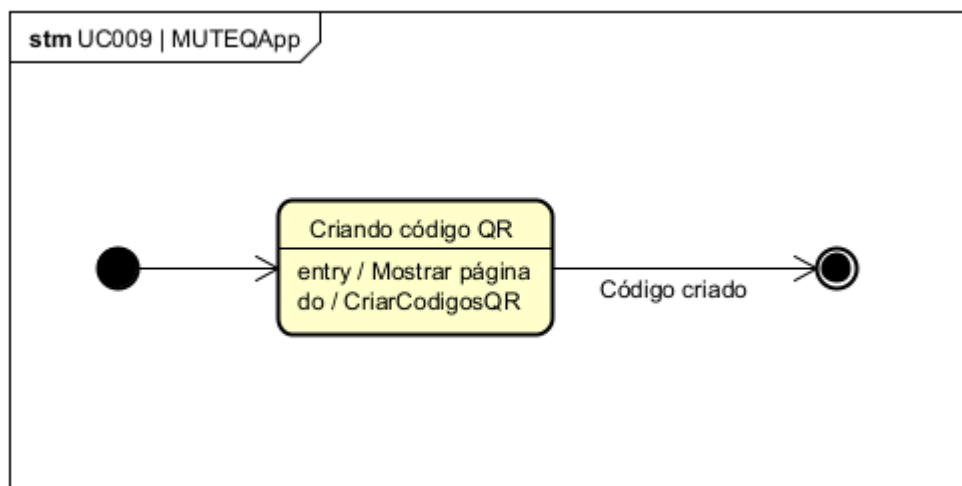
Figura 82. Diagrama de Estados da classe MUTEQApp para o [UC009].
