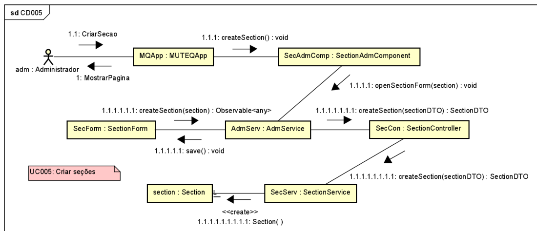
Figura 51. Diagrama de comunicação para o [UC005].
