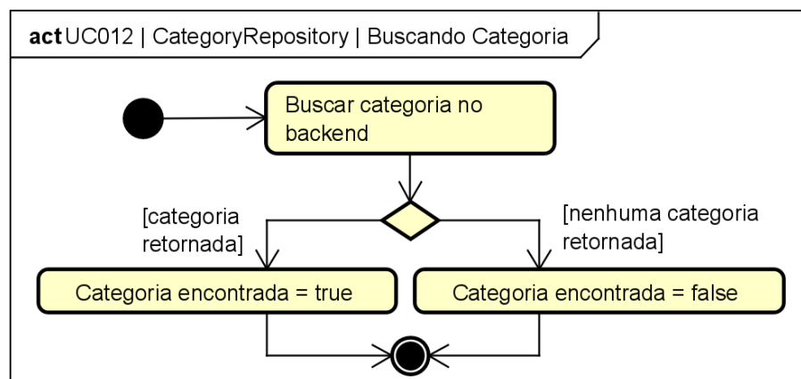
Figura 122. Diagrama de Atividades do estado “Buscando Categoria” da classe CategoryRespository para o [UC012].
