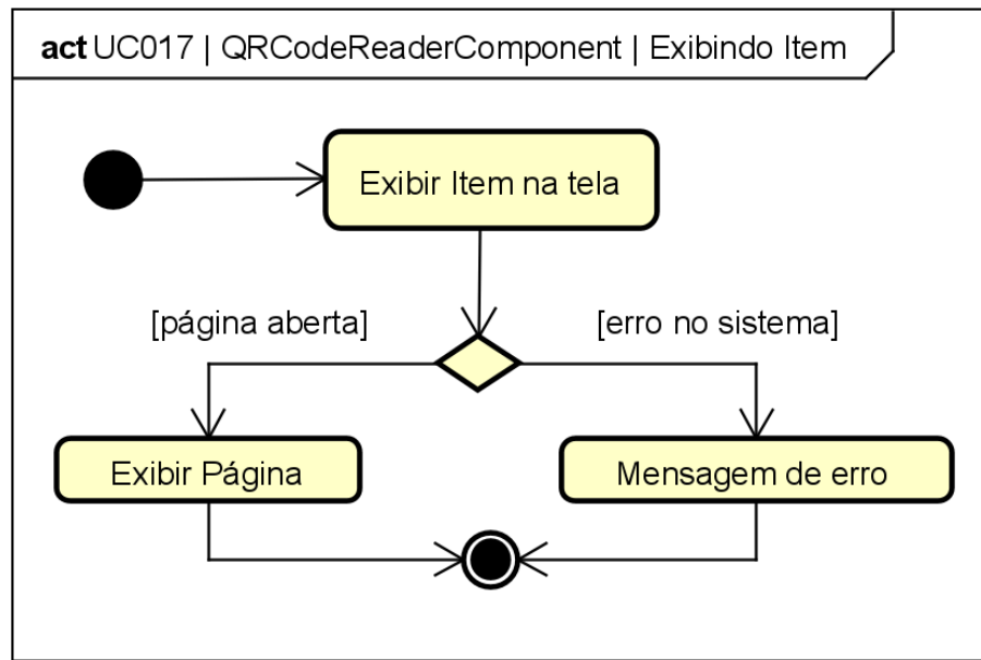
Figura 131. Diagrama de Atividades do estado “Exibindo Item” da classe QRCodeReaderComponent para o [UC017].
