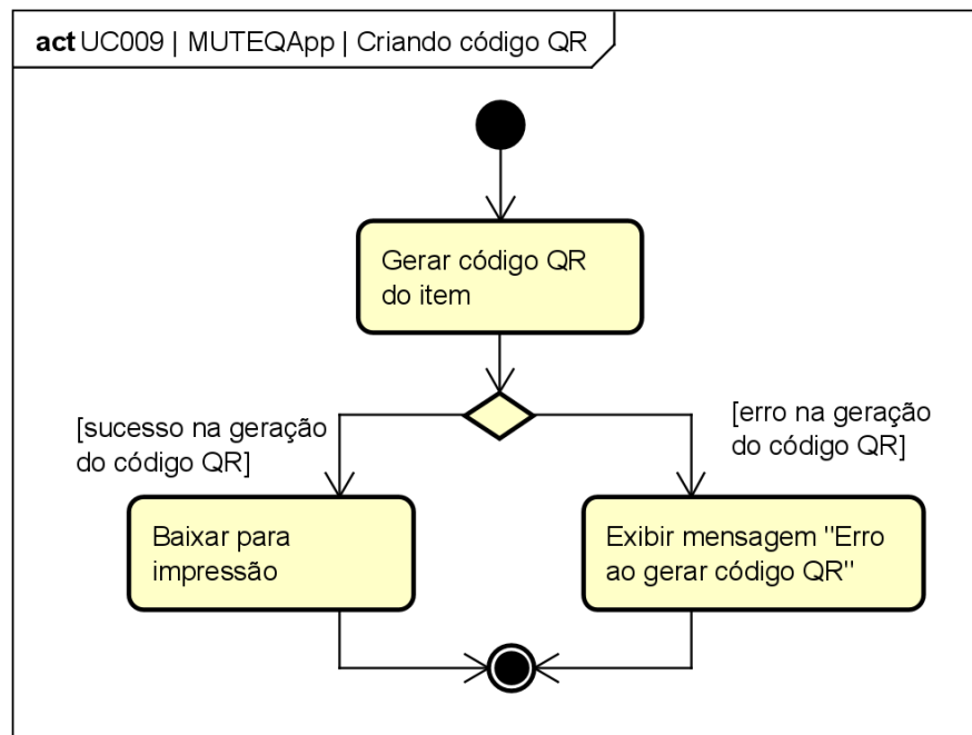
Figura 116. Diagrama de Atividades do estado “Criando código QR” da classe MUTEQApp para o [UC009].
