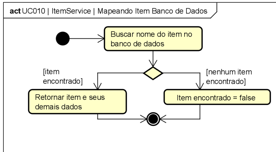
Figura 117. Diagrama de Atividades do estado “Mapeando Item Banco de Dados” da classe ItemService para o [UC010].
