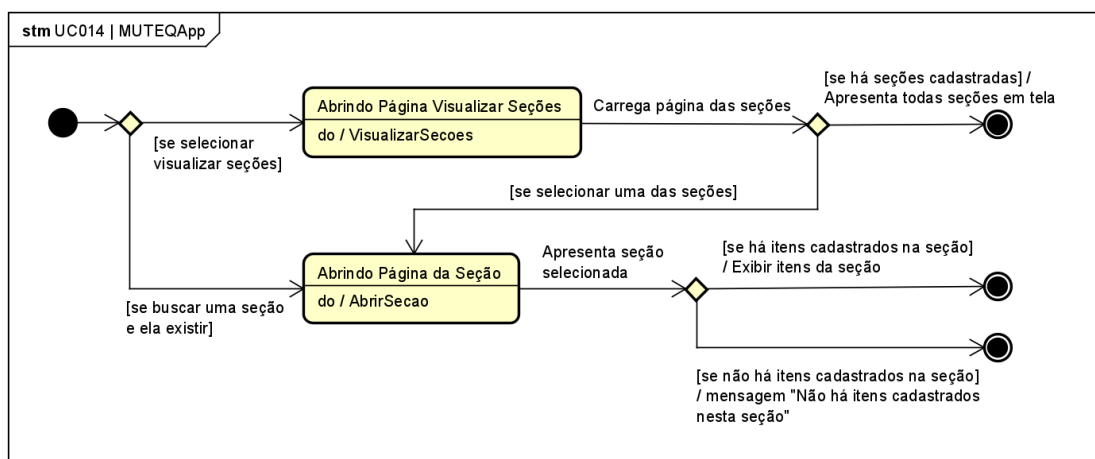
Figura 91. Diagrama de Estados da classe MUTEQApp para o [UC014].
