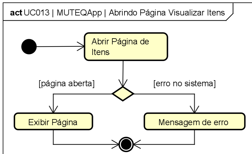
Figura 124. Diagrama de Atividades do estado “Abrindo Página Visualizar Itens” da classe MUTEQApp para o [UC013].
