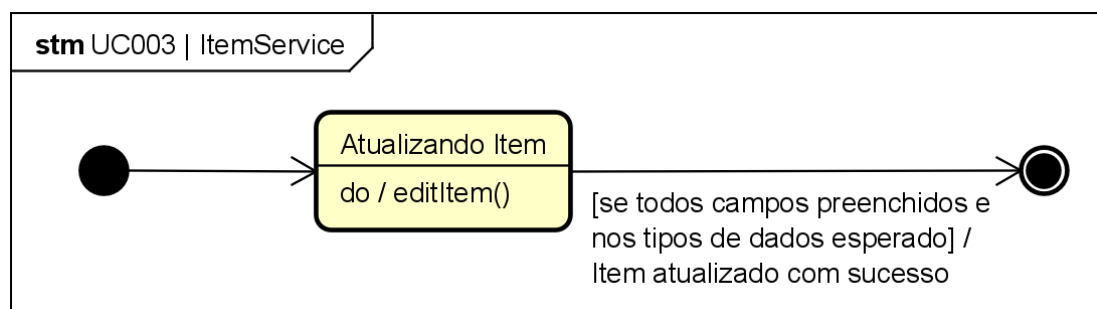
Figura 70. Diagrama de Estados da classe ItemService para o [UC003].
