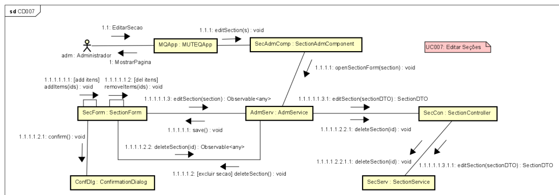
Figura 53. Diagrama de comunicação para o [UC007].
