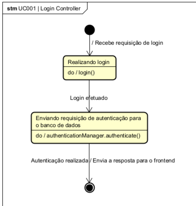
Figura 66. Diagrama de Estados da classe LoginController para o [UC001].
