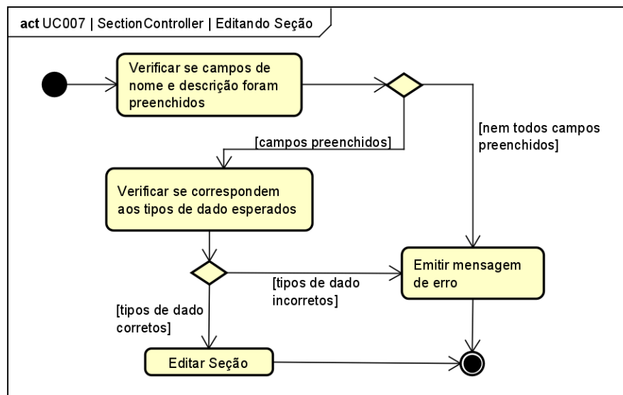
Figura 112. Diagrama de Atividades do estado “Editando Seção” da classe SectionController para o [UC007].
