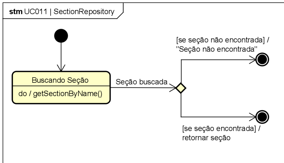
Figura 86. Diagrama de Estados da classe SectionRepository para o [UC011].
