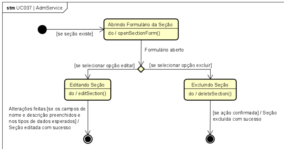
Figura 77. Diagrama de Estados da classe AdmService para o [UC007].
