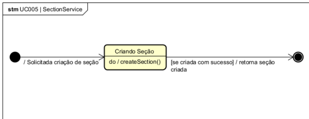
Figura 74. Diagrama de Estados da classe SectionService para o [UC005].
