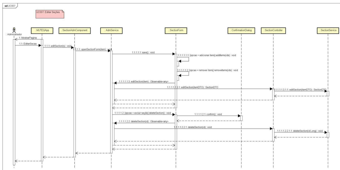
Figura 36. Diagrama de sequência para o [UC007].
