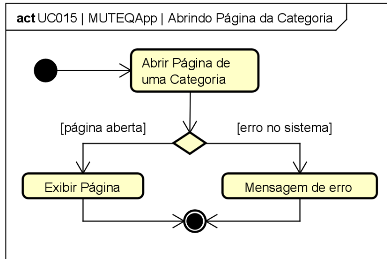
Figura 127. Diagrama de Atividades do estado “Abrindo Página da Categoria” da classe MUTEQApp para o [UC015].
