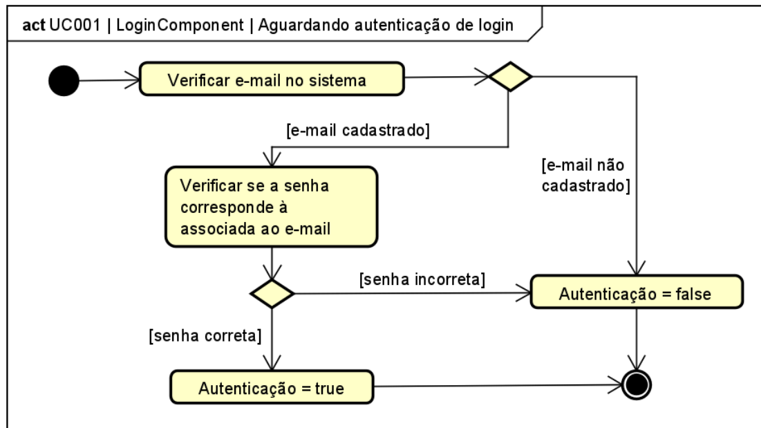
Figura 99. Diagrama de Atividades do estado “Aguardando autenticação de login” da classe LoginComponent para o [UC001].
