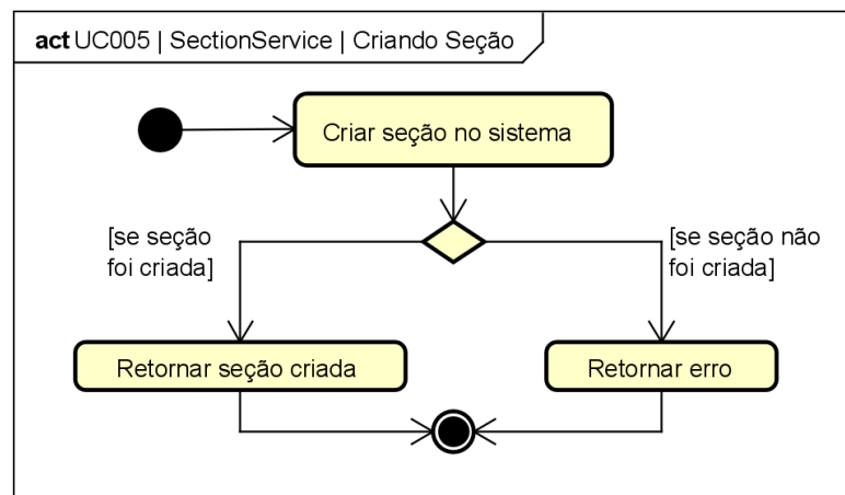
Figura 108. Diagrama de Atividades do estado “Criando seção” da classe SectionService para o [UC005].
