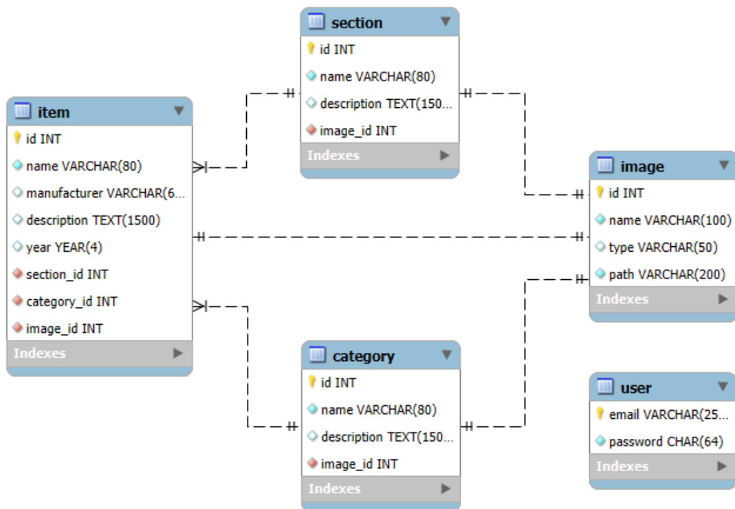
Figura 64. Diagrama Entidade-Relacionamento (DER).
