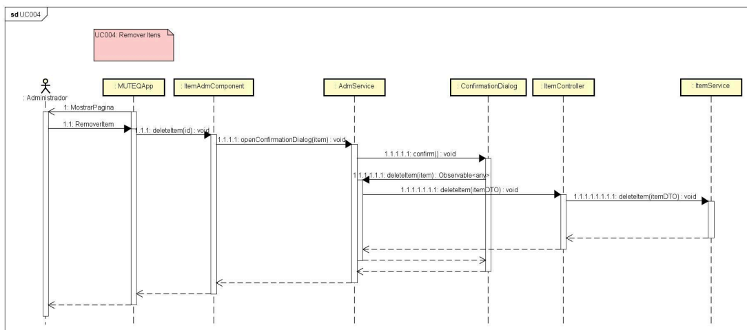
Figura 33. Diagrama de sequência para o [UC004].
