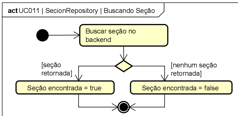
Figura 120. Diagrama de Atividades do estado “Buscando Seção” da classe SectionRespository para o [UC011].
