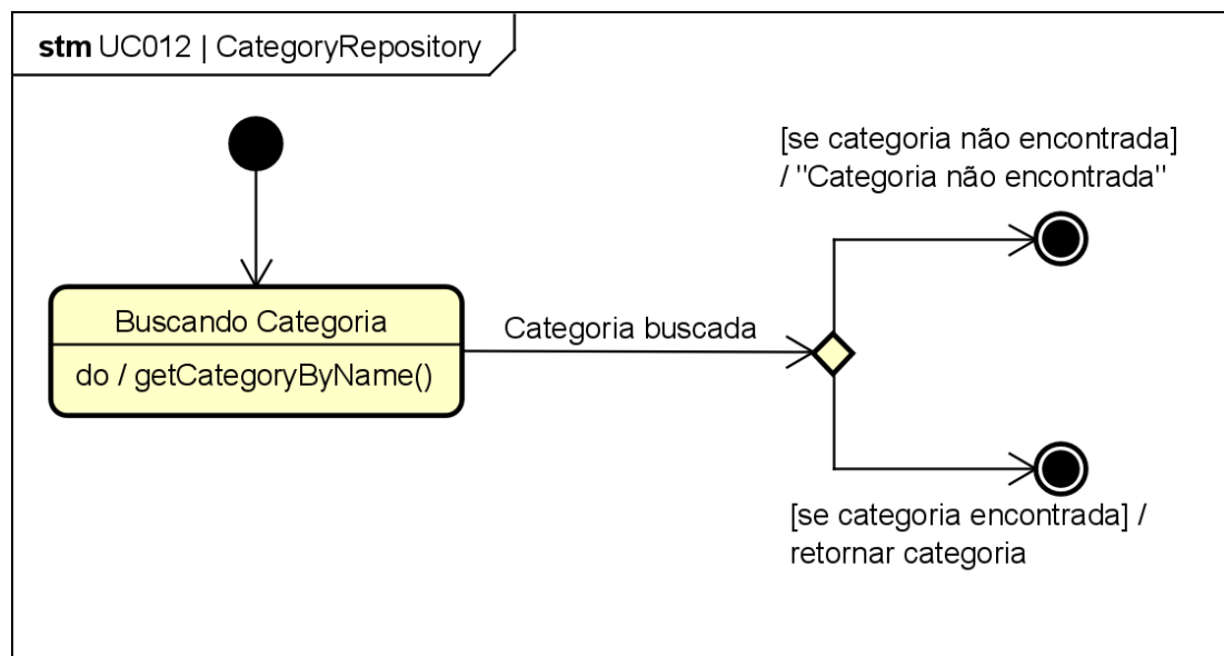
Figura 88. Diagrama de Estados da classe CategoryRepository para o [UC012].
