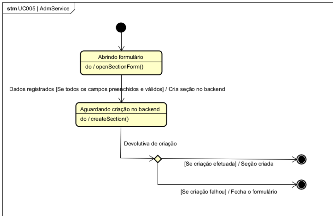
Figura 73. Diagrama de Estados da classe AdmService para o [UC005].
