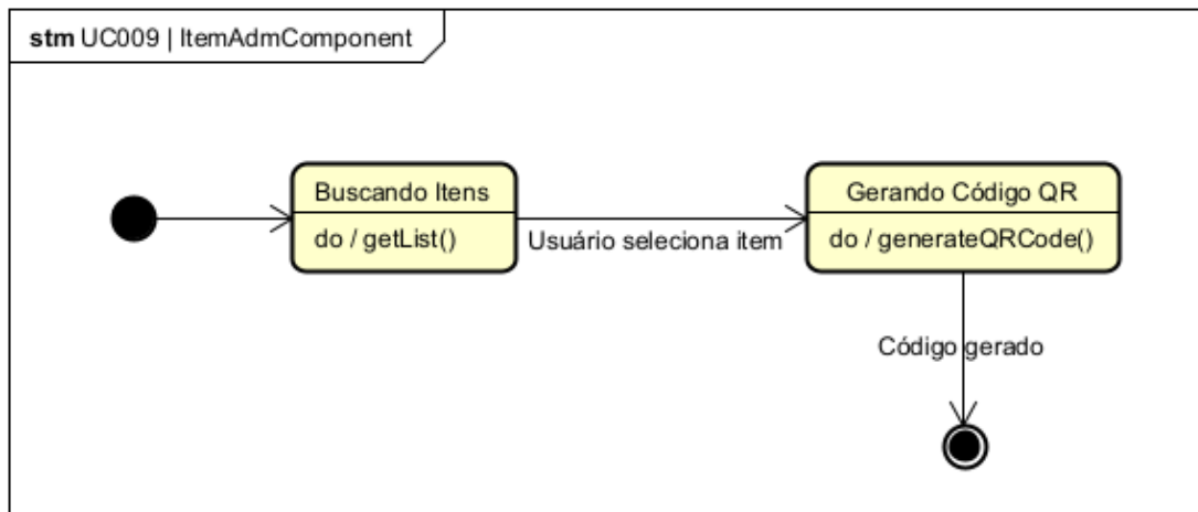
Figura 81. Diagrama de Estados da classe ItemAdmComponent para o [UC009].
