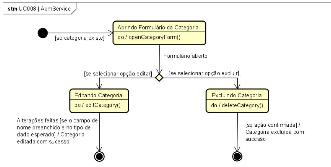
Figura 79. Diagrama de Estados da classe AdmService para o [UC008].
