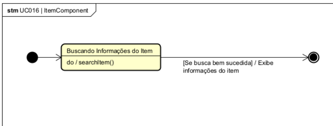
Figura 96. Diagrama de Estados da classe ItemComponent para o [UC016].
