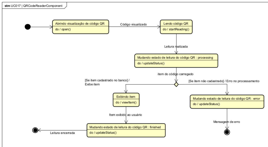
Figura 97. Diagrama de Estados da classe QRCodeReaderComponent para o [UC017].
