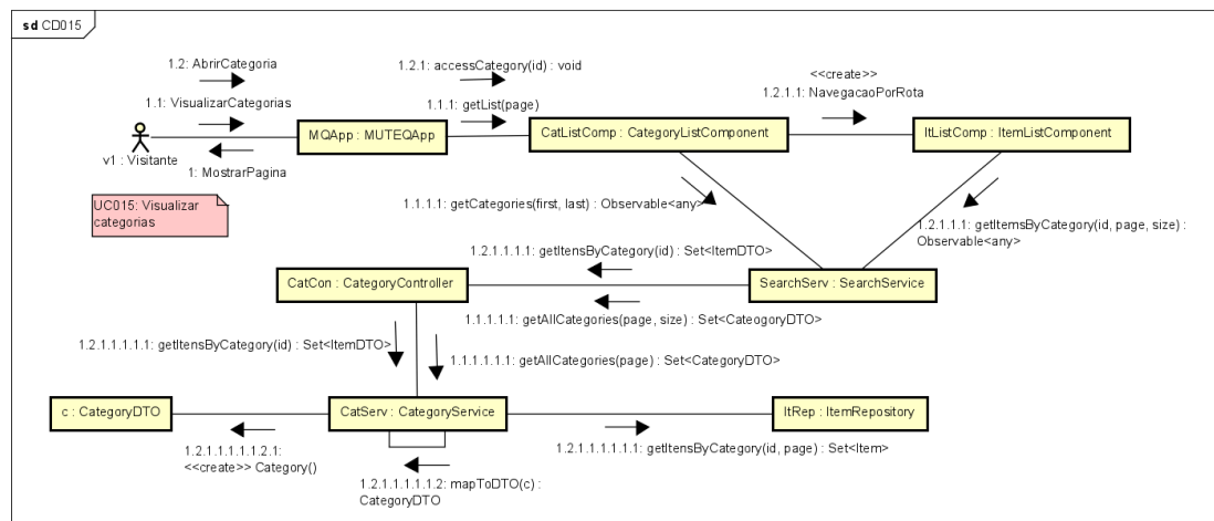
Figura 61. Diagrama de comunicação para o [UC015].
