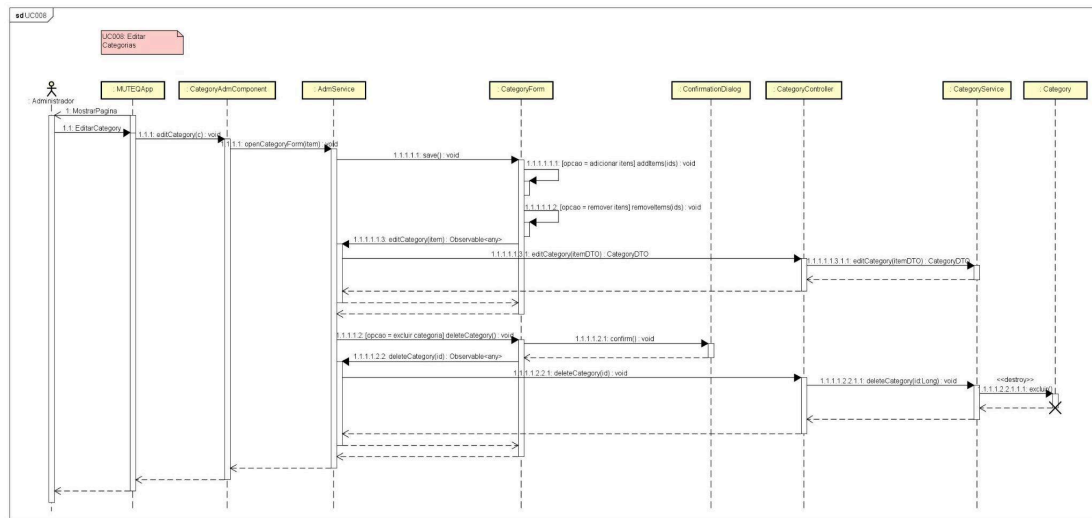
Figura 37. Diagrama de sequência para o [UC008].
