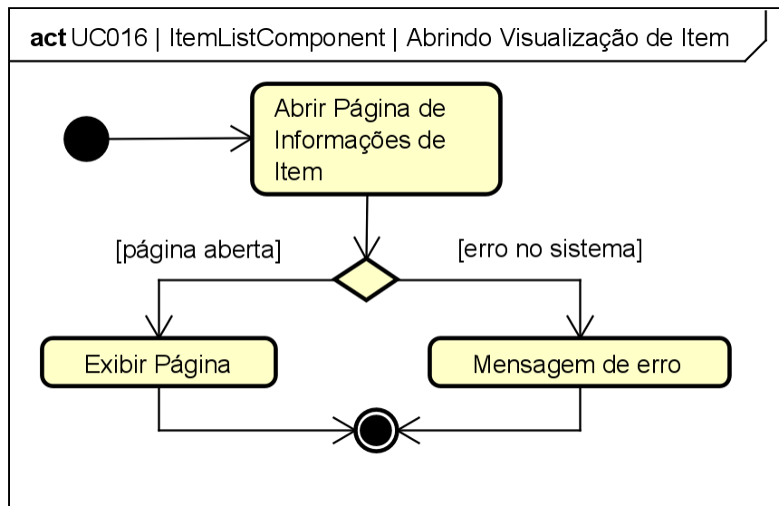
Figura 129. Diagrama de Atividades do estado “Abrindo Visualização de Item” da classe ItemListComponent para o [UC016].
