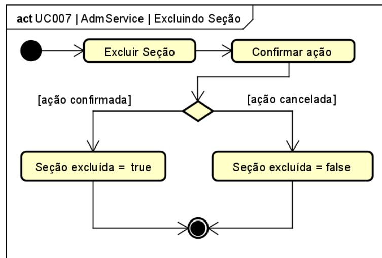
Figura 111. Diagrama de Atividades do estado “Excluindo Seção” da classe AdmService para o [UC007].
