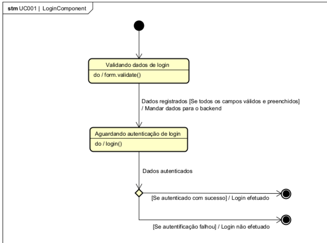
Figura 65. Diagrama de Estados da classe LoginComponent para o [UC001].
