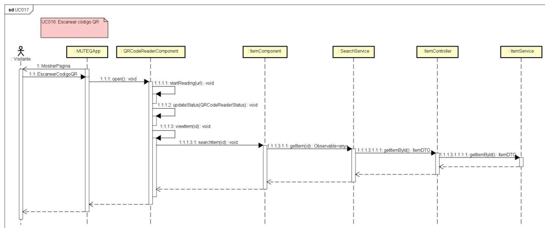
Figura 46. Diagrama de sequência para o [UC017].
