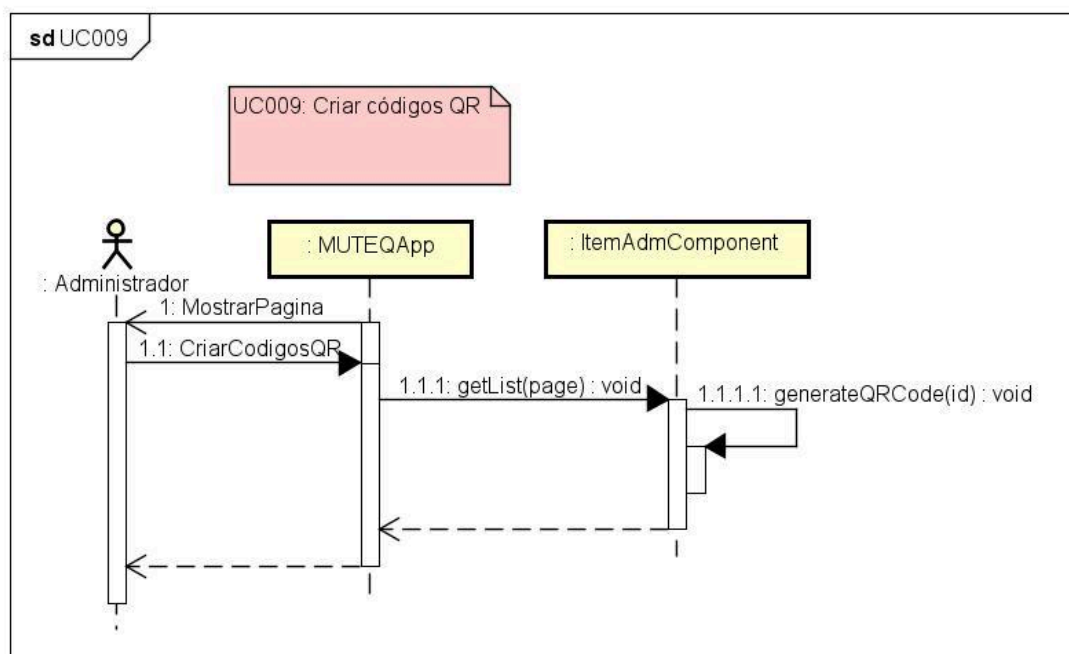
Figura 38. Diagrama de sequência para o [UC009].
