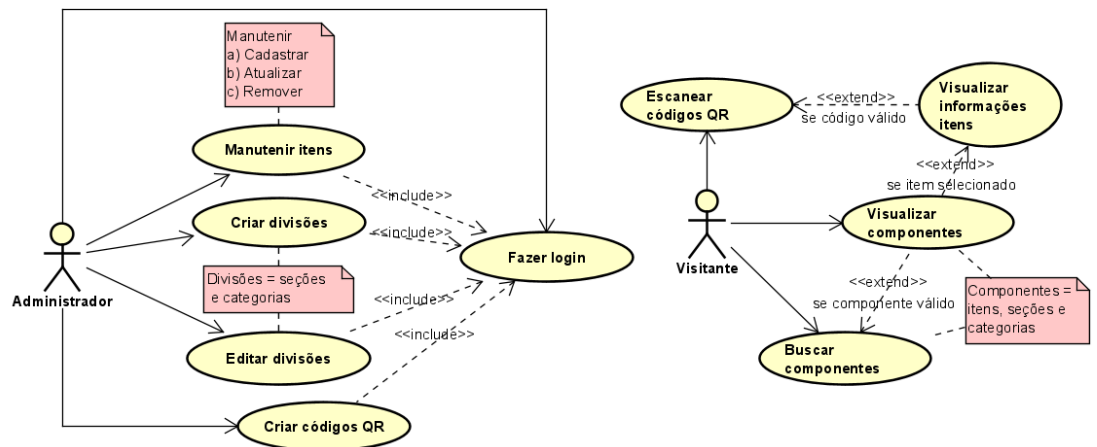
Figura 19. Diagrama de casos de uso.
