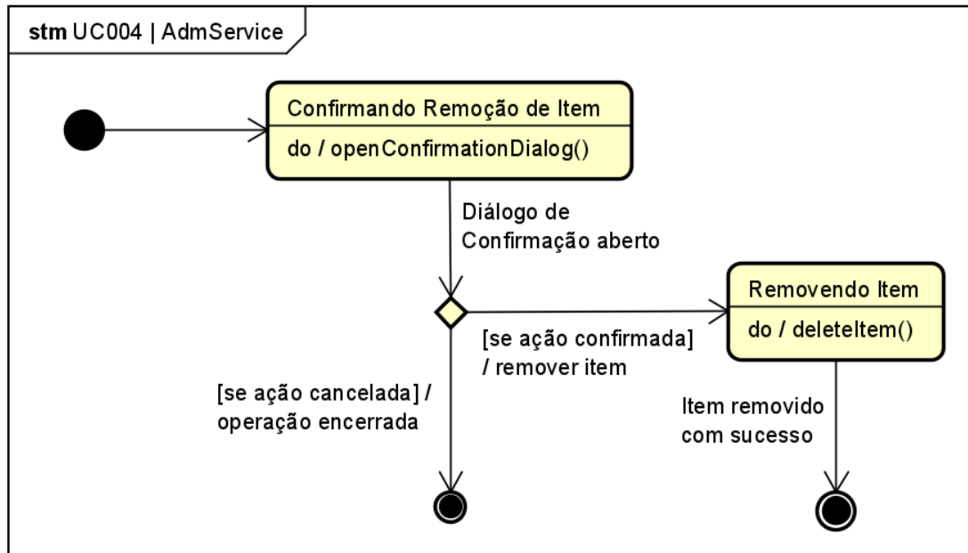
Figura 71. Diagrama de Estados da classe AdmService para o [UC004].
