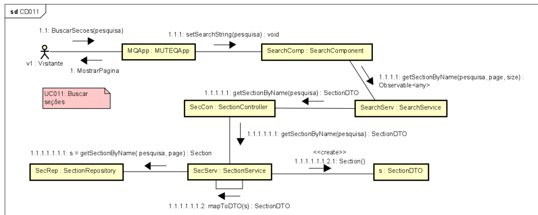
Figura 57. Diagrama de comunicação para o [UC011].
