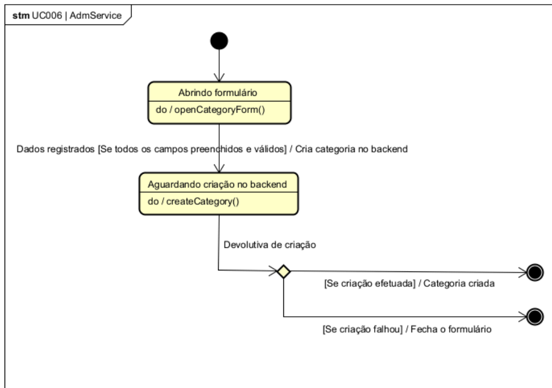
Figura 75. Diagrama de Estados da classe AdmService para o [UC006].
