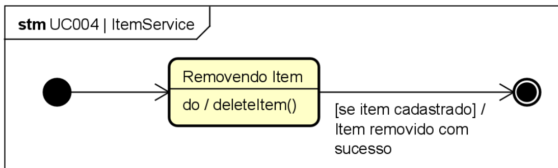
Figura 72. Diagrama de Estados da classe ItemService para o [UC004].
