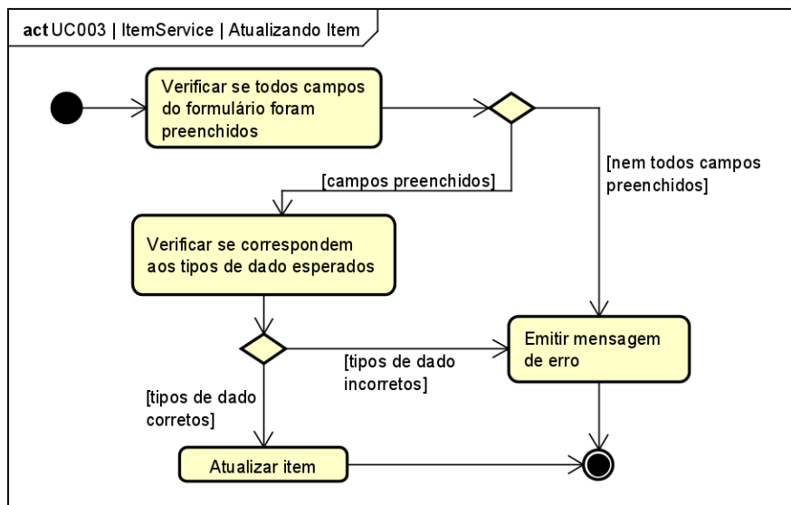
Figura 104. Diagrama de Atividades do estado “Atualizando Item” da classe ItemService para o [UC003].
