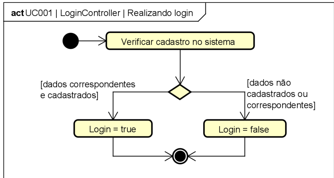
Figura 100. Diagrama de Atividades do estado “Realizando login” da classe LoginController para o [UC001].
