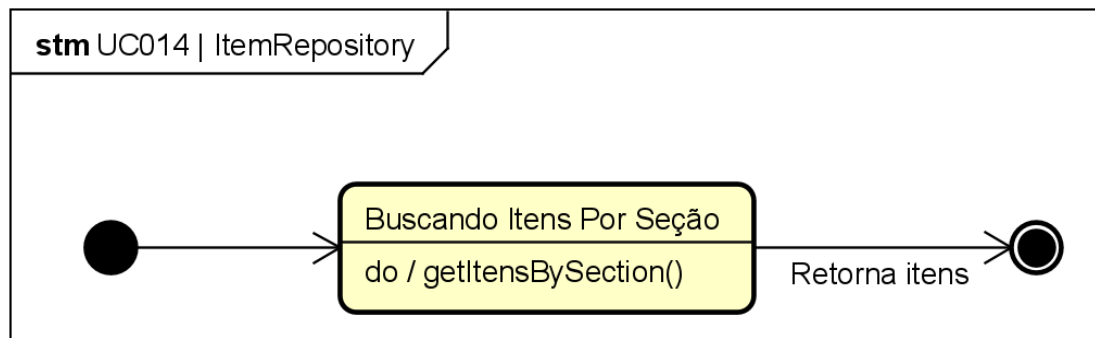
Figura 92. Diagrama de Estados da classe ItemRepository para o [UC014].
