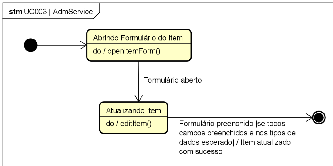
Figura 69. Diagrama de Estados da classe AdmService para o [UC003].
