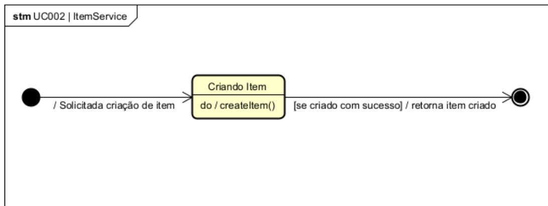
Figura 68. Diagrama de Estados da classe ItemService para o [UC002].
