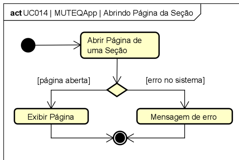
Figura 125. Diagrama de Atividades do estado “Abrindo Página da Seção” da classe MUTEQApp para o [UC014].
