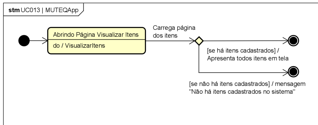
Figura 90. Diagrama de Estados da classe MUTEQApp para o [UC013].
