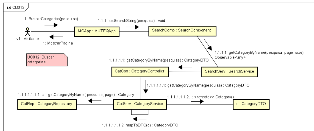
Figura 58. Diagrama de comunicação para o [UC012].
