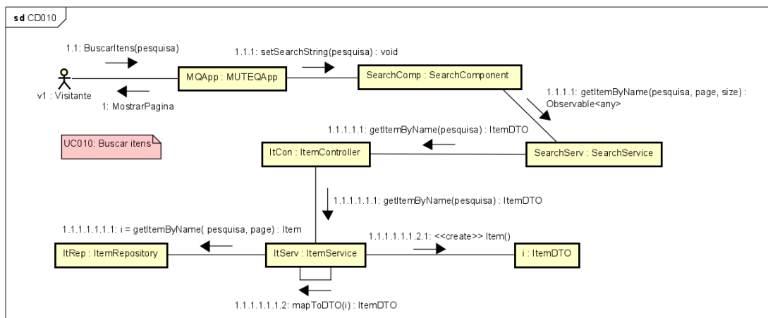
Figura 56. Diagrama de comunicação para o [UC010].
