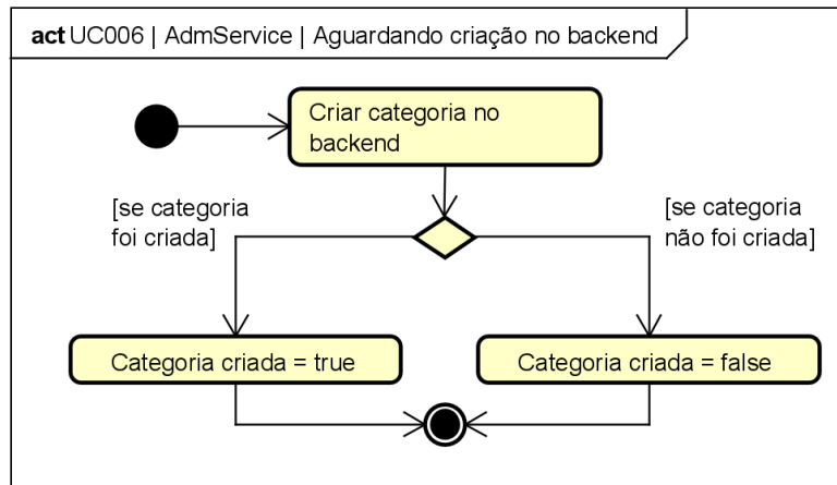
Figura 109. Diagrama de Atividades do estado “Aguardando criação no backend” da classe AdmService para o [UC006].
