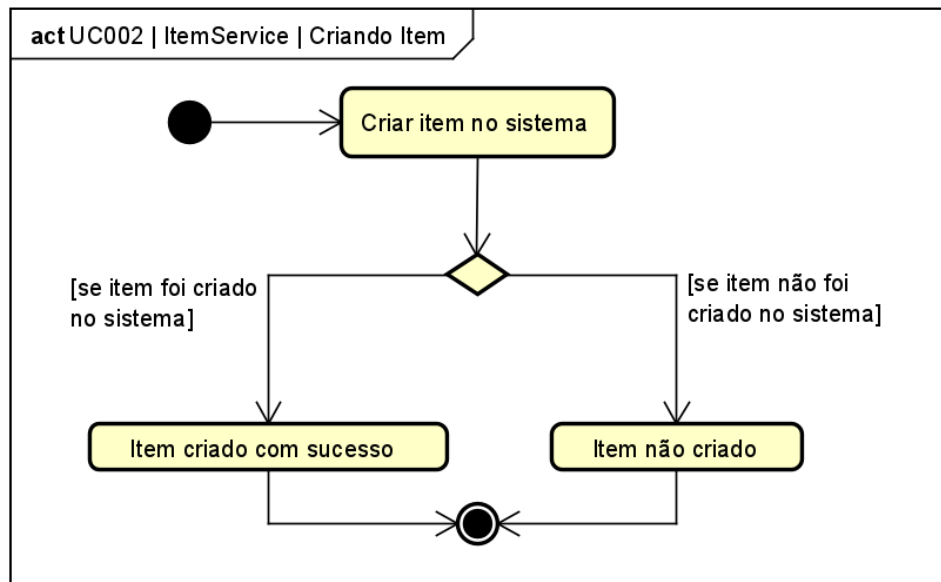
Figura 102. Diagrama de Atividades do estado “Criando Item” da classe ItemService para o [UC002].
