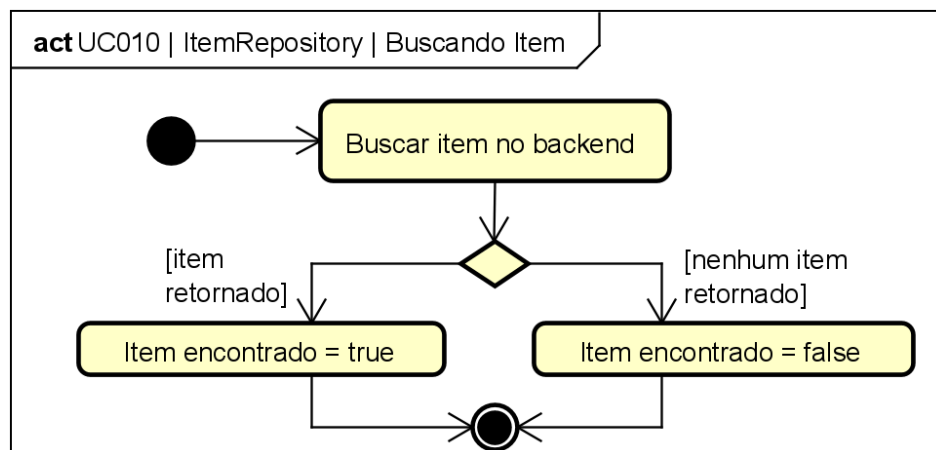
Figura 118. Diagrama de Atividades do estado “Buscando Item” da classe ItemRepository para o [UC010].
