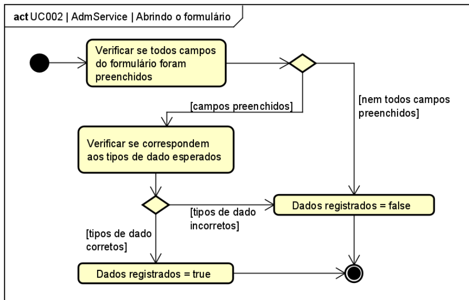
Figura 101. Diagrama de Atividades do estado “Abrindo o formulário” da classe AdmService para o [UC002].
