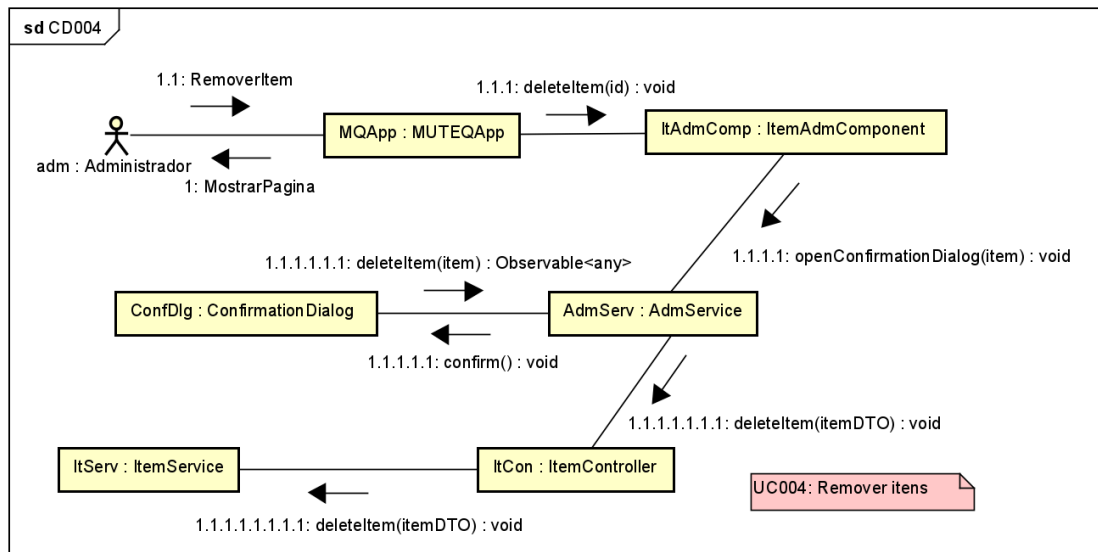
Figura 50. Diagrama de comunicação para o [UC004].
