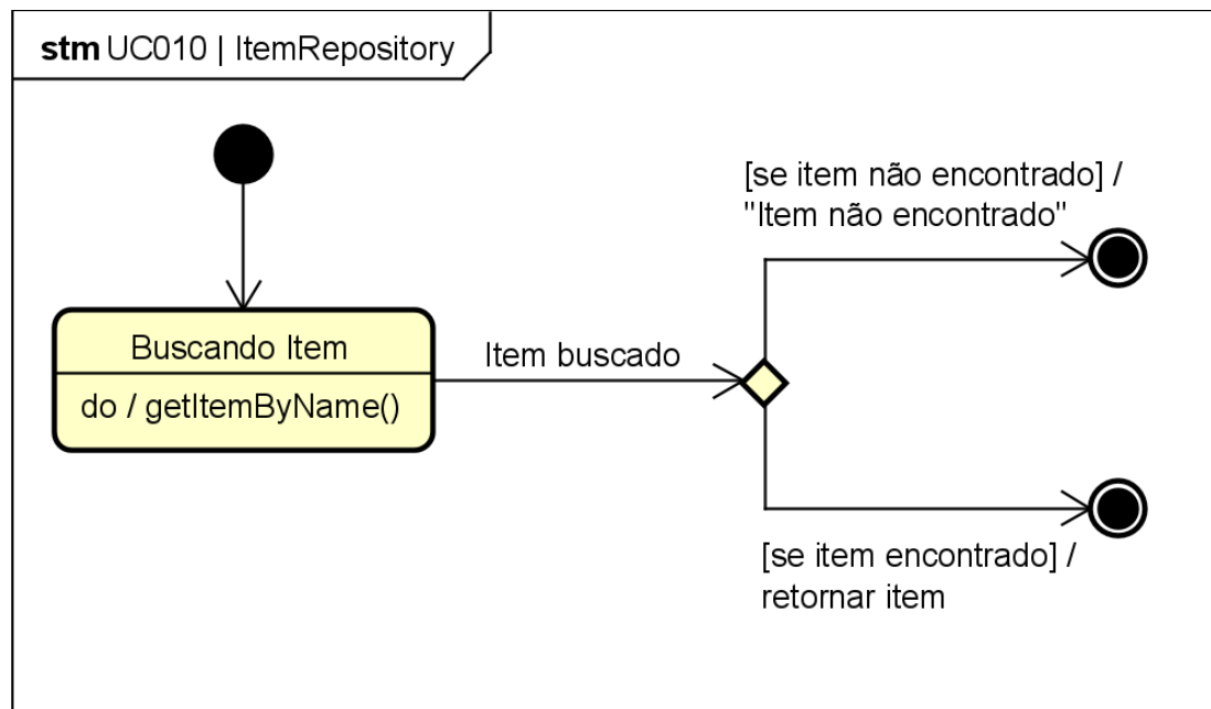
Figura 84. Diagrama de Estados da classe ItemRepository para o [UC010].
