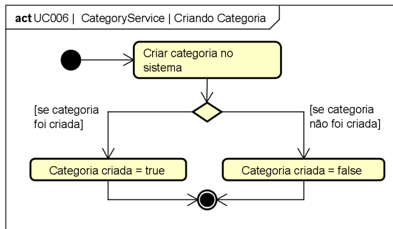
Figura 110. Diagrama de Atividades do estado “Criando Categoria” da classe CategoryService para o [UC006].
