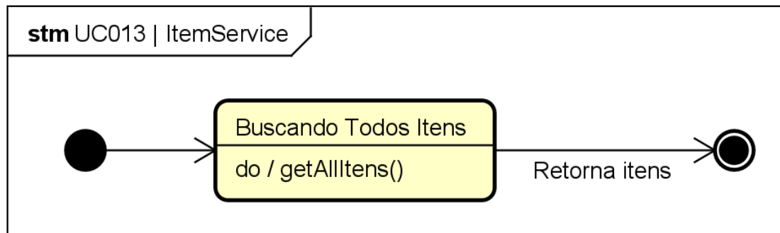
Figura 89. Diagrama de Estados da classe ItemService para o [UC013].
