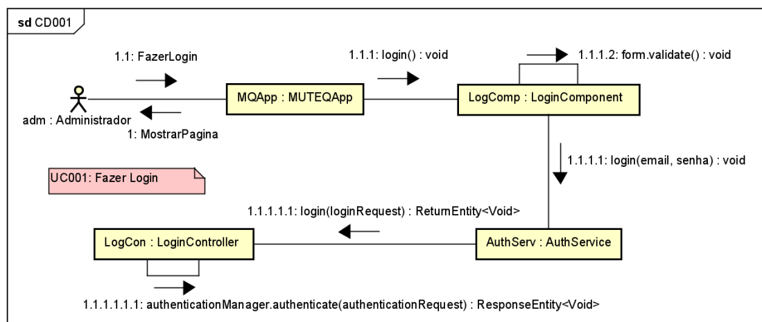
Figura 47. Diagrama de comunicação para o [UC001].
