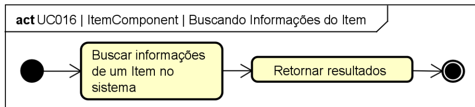
Figura 130. Diagrama de Atividades do estado “Buscando Informações do Item” da classe ItemComponent para o [UC016].
