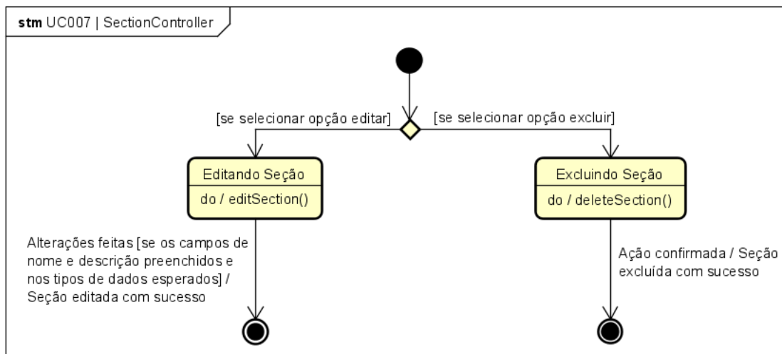
Figura 78. Diagrama de Estados da classe SectionController para o [UC007].
