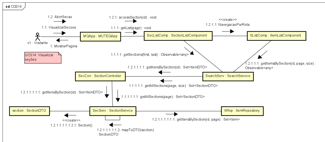
Figura 60. Diagrama de comunicação para o [UC014].
