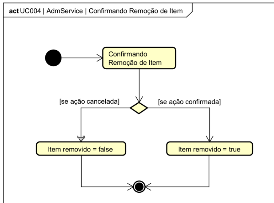
Figura 105. Diagrama de Atividades do estado “Confirmando Remoção de Item” da classe AdmService para o [UC004].
