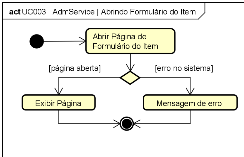
Figura 103. Diagrama de Atividades do estado “Abrindo Formulário do Item” da classe AdmService para o [UC003].
