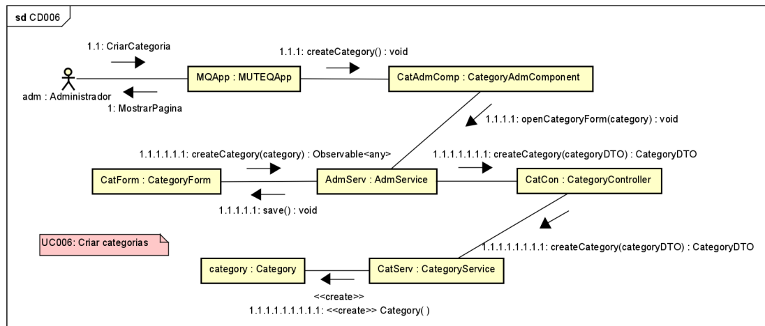
Figura 52. Diagrama de comunicação para o [UC006].
