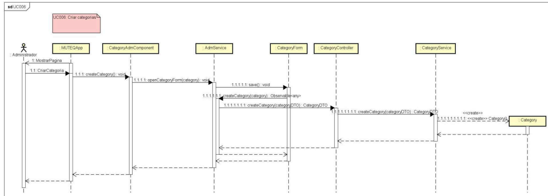
Figura 35. Diagrama de sequência para o [UC006].
