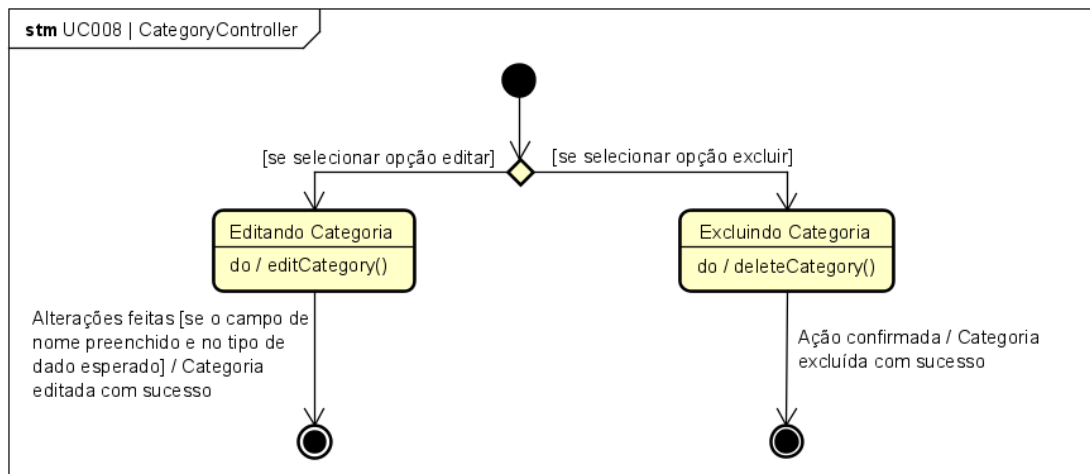
Figura 80. Diagrama de Estados da classe CategoryController para o [UC008].
