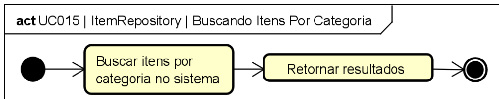
Figura 128. Diagrama de Atividades do estado “Buscando Itens Por Categoria” da classe ItemRepository para o [UC015].
