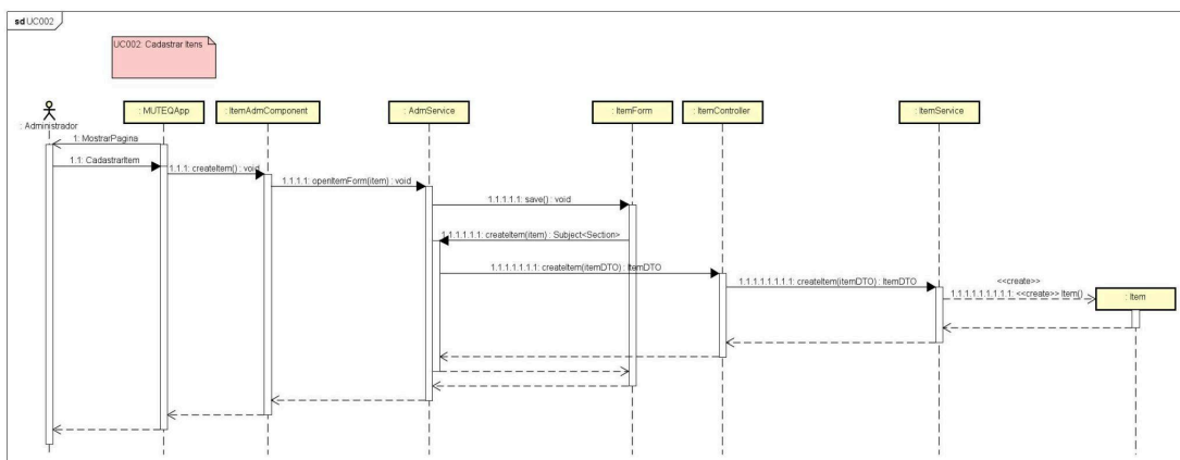
Figura 31. Diagrama de sequência para o [UC002].
