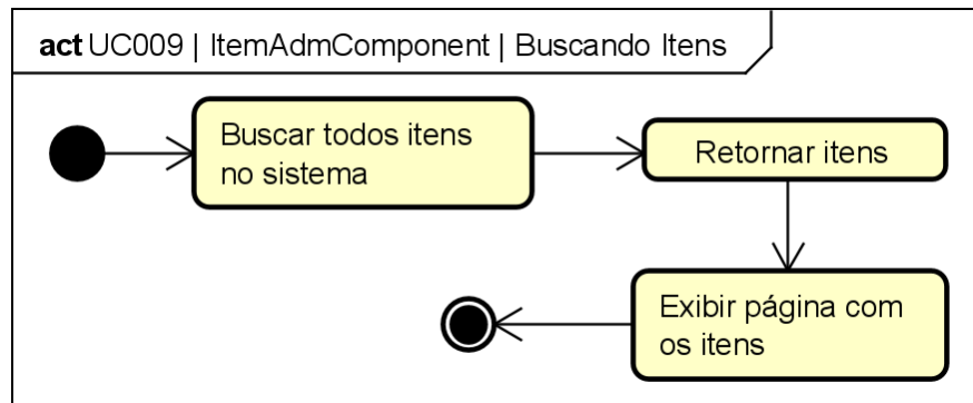
Figura 115. Diagrama de Atividades do estado “Buscando itens” da classe ItemAdmComponent para o [UC009].
