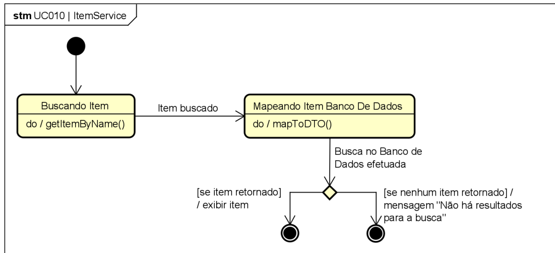
Figura 83. Diagrama de Estados da classe ItemService para o [UC010].
