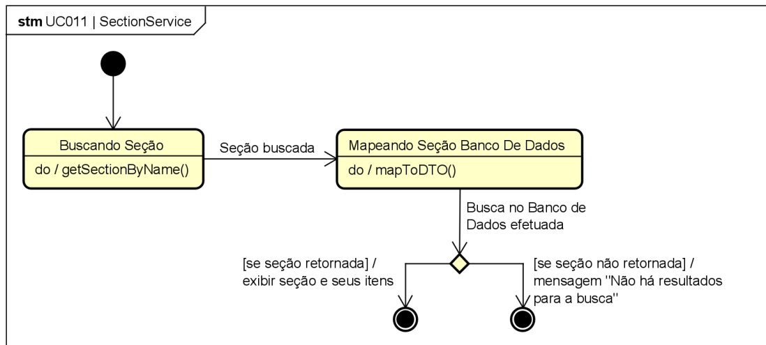
Figura 85. Diagrama de Estados da classe SectionService para o [UC011].
