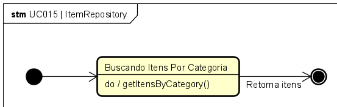
Figura 94. Diagrama de Estados da classe ItemRepository para o [UC015].
