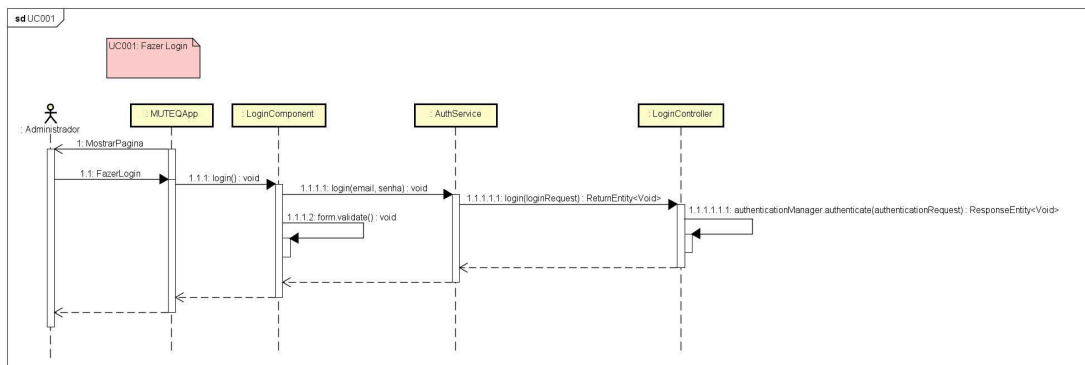
Figura 30. Diagrama de sequência para o [UC001].
