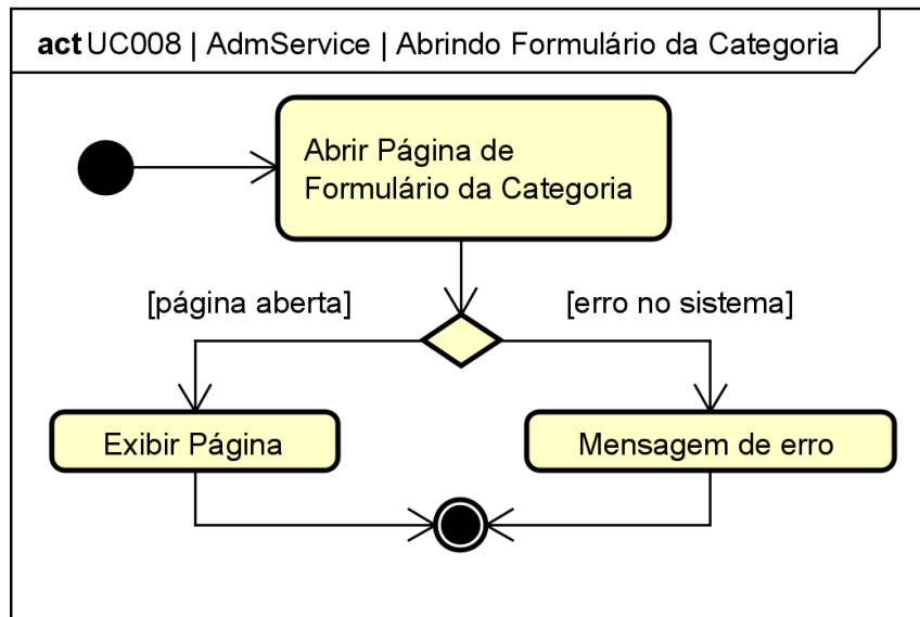
Figura 113. Diagrama de Atividades do estado “Abrindo Formulário da Categoria” da classe AdmService para o [UC008].
