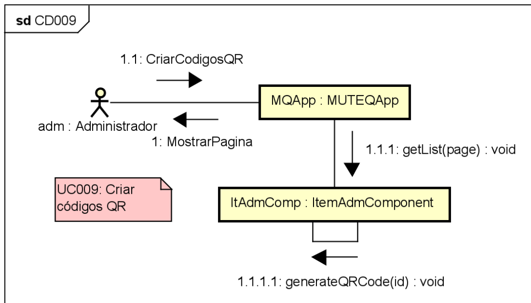
Figura 55. Diagrama de comunicação para o [UC009].
