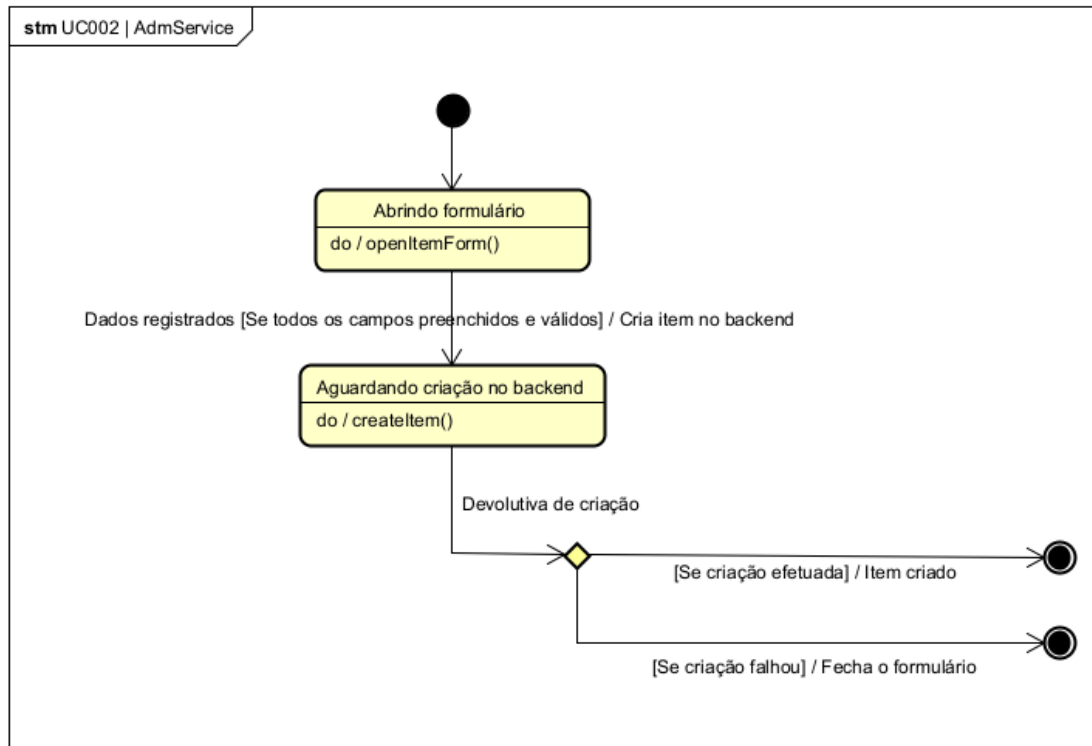
Figura 67. Diagrama de Estados da classe AdmService para o [UC002].
