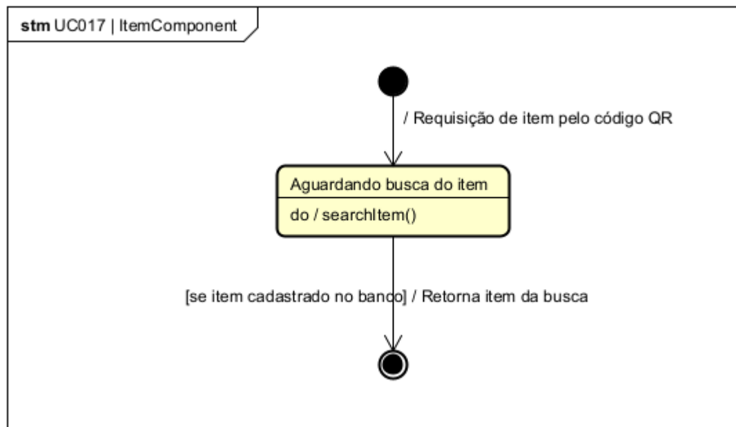
Figura 98. Diagrama de Estados da classe ItemComponent para o [UC017].
