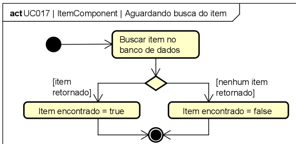
Figura 132. Diagrama de Atividades do estado “Aguardando Busca do Item” da classe ItemComponent para o [UC017].
