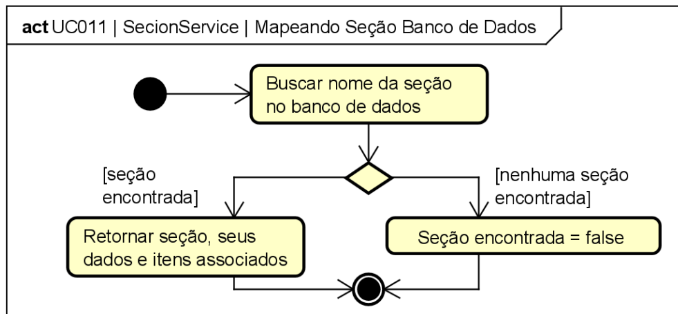
Figura 119. Diagrama de Atividades do estado “Mapeando Seção Banco de Dados” da classe SectionService para o [UC011].
