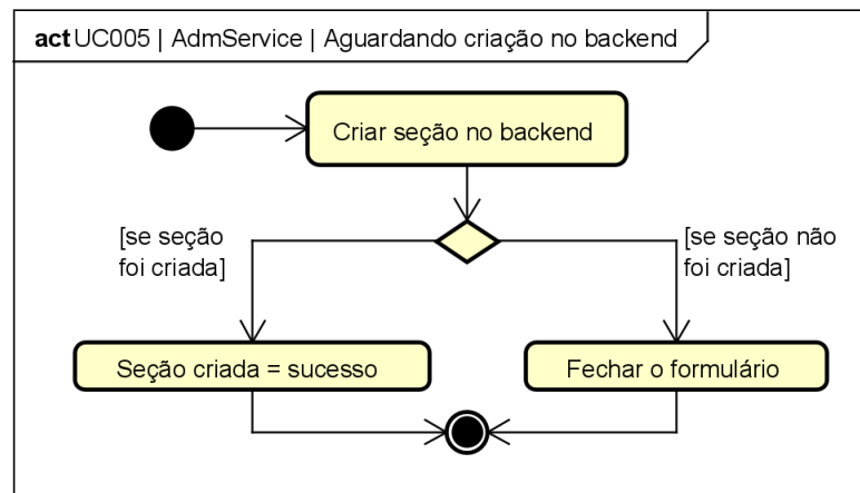
Figura 107. Diagrama de Atividades do estado “Aguardando criação no backend” da classe AdmService para o [UC005].
