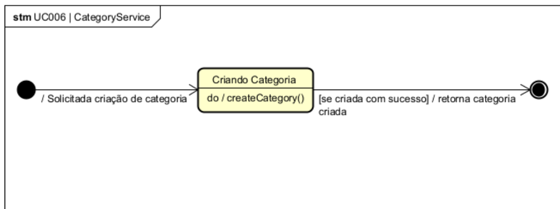
Figura 76. Diagrama de Estados da classe CategoryService para o [UC006].
