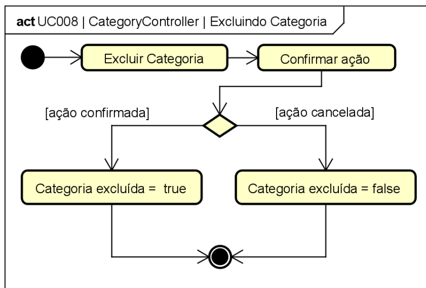
Figura 114. Diagrama de Atividades do estado “Excluindo Categoria” da classe CategoryController para o [UC008].
