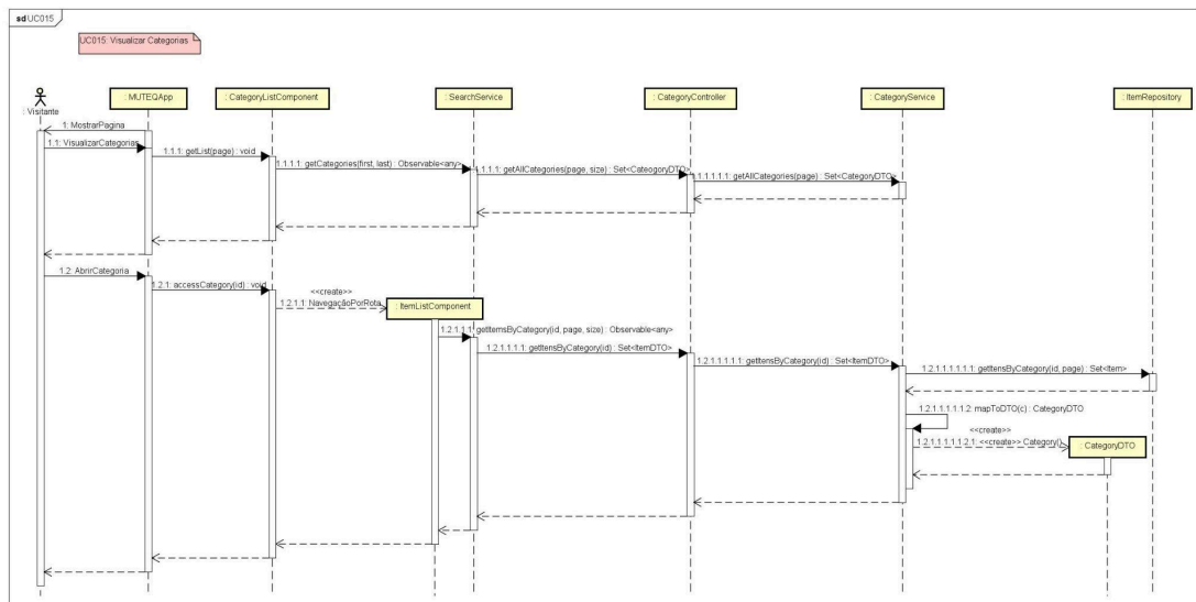
Figura 44. Diagrama de seqüência para o [UC015].
