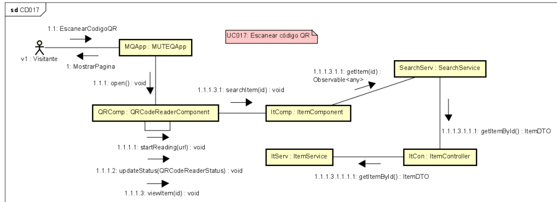
Figura 63. Diagrama de comunicação para o [UC017].
