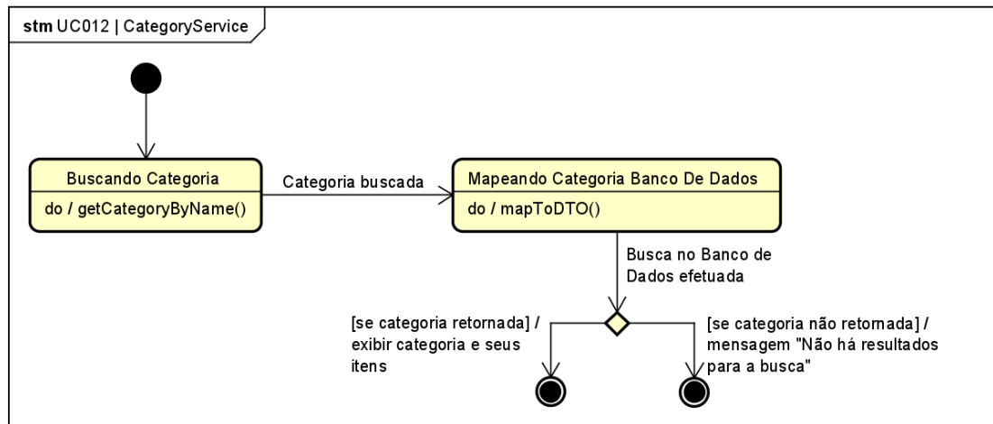
Figura 87. Diagrama de Estados da classe CategoryService para o [UC012].
